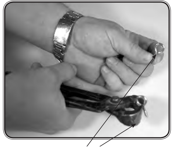
❶ Ringschraube mit Beißzange öffnen
