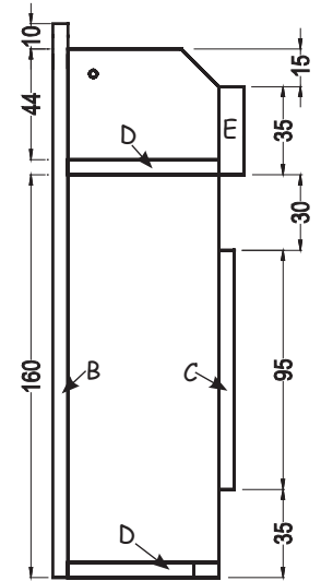
Schnitt - Mitte
